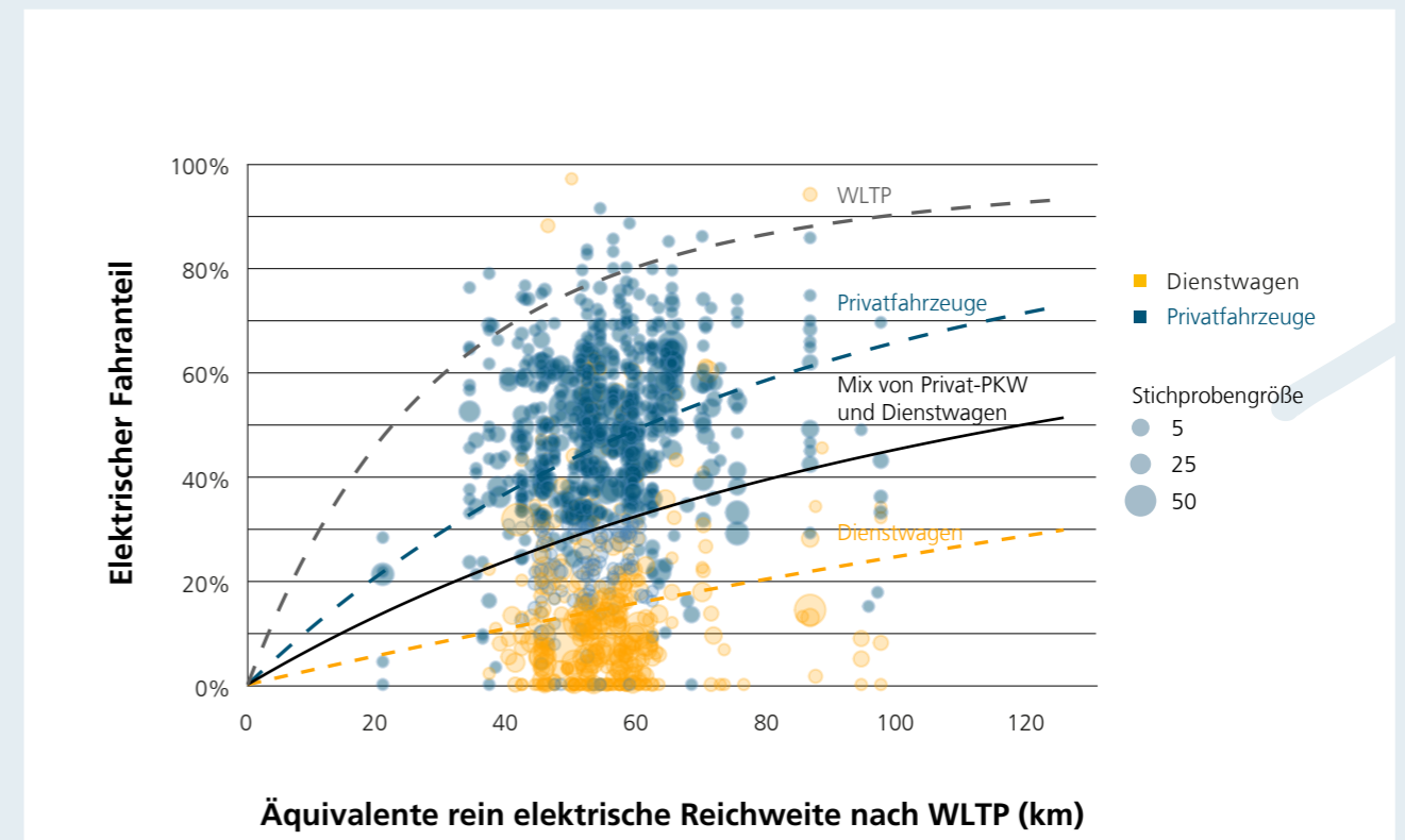
Abbildung 2. Realer elektrischer Fahranteil im Vergleich zu den WLTP-Annahmen über den Fahranteil im Charge-Depleting -Modus.
