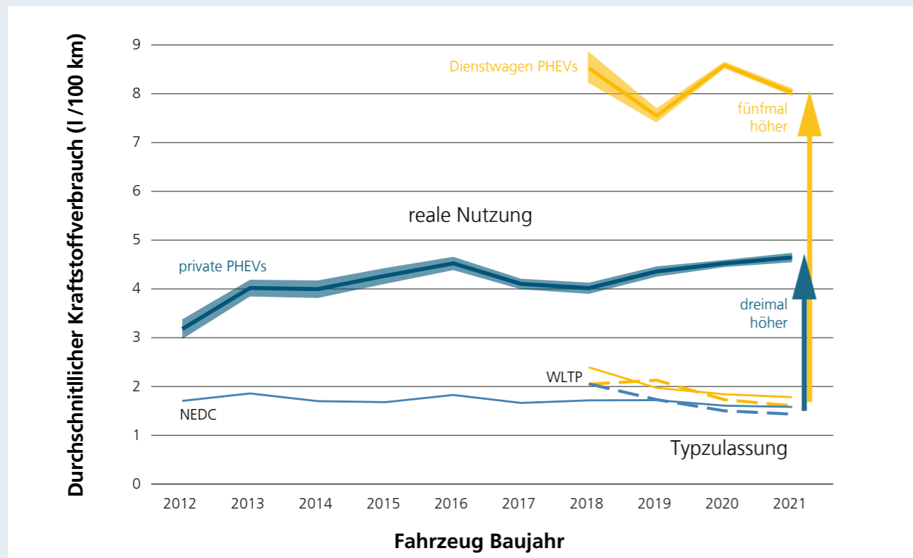
Abbildung 1. Entwicklung des durchschnittlichen realen und offiziellen Kraftstoffverbrauchs von als Privat- und als Dienstwagen genutzten PHEV in Europa über das Baujahr der Fahrzeuge. Die schattierten Bereiche stellen das 95 Prozent-Konfidenzintervall der Stichprobenmittelwerte dar.
